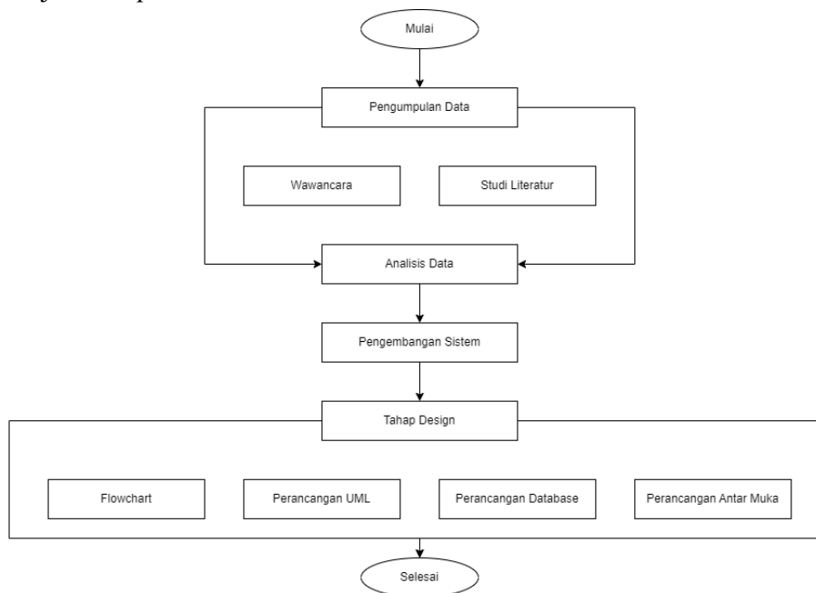
Gambar 1. Jalan penelitian
